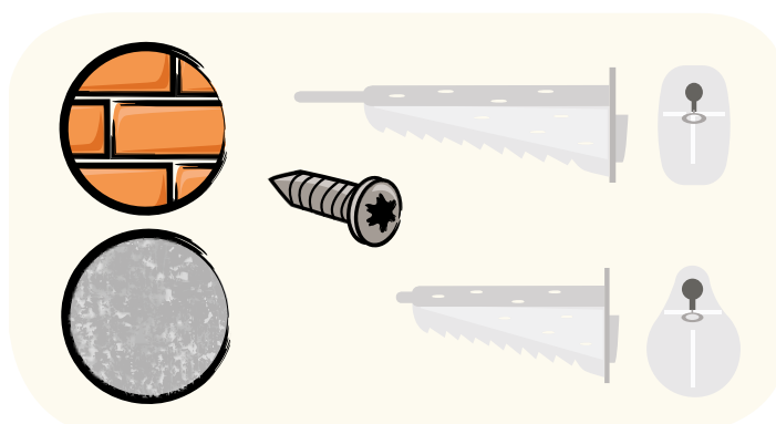
3. C webertherm 317 + webertherm 312 fäste MTB / webertherm 312 fäste TB
