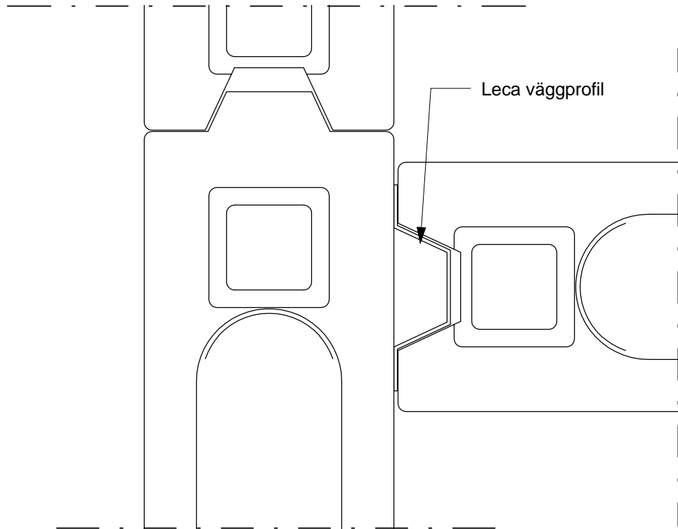
Detalj skala 1:2
